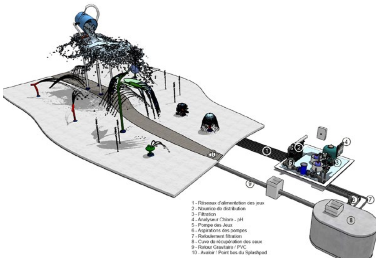
© Schéma du système de filtration en eau recyclée - Propriété AQUA PRO URBA
